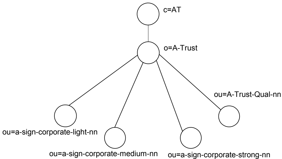
Abbildung 2 a.trust Verzeichnisbaum
